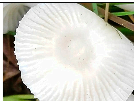
CUPHOPHYLLUS VIRGINEUS, STRIATURA
